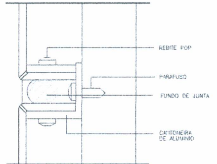
CORTE VERTICAL ESC.: 1:5
