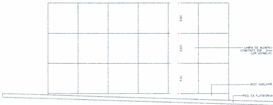
VISTA B ESC.: 1:30
