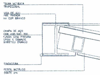
DETALHE 07 esc.: 1:5
