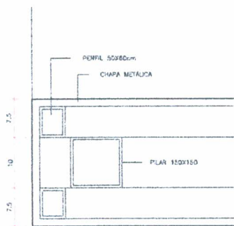
DETALHE 05 esc.: 1:5
