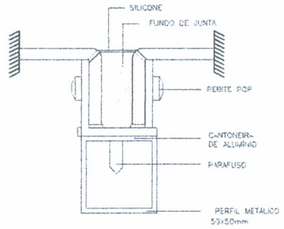
CORTE HORIZONTAL ESC.: 1:5
