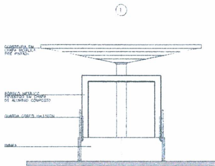
VISTA C esc.: 1:50
