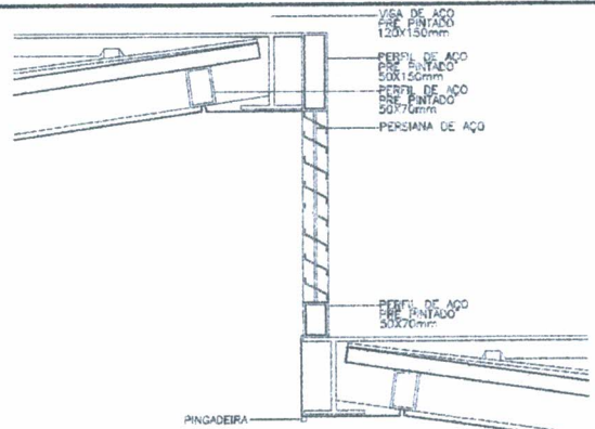
DETALHE 06 esc.: 1:5
